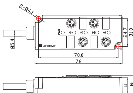
S010-M8-4/4P/4C
