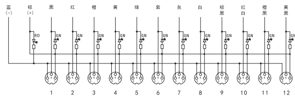
S010-M8-12 S011-M8-12
