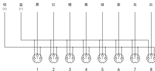
S010-M8-8C S011-M8-8C
