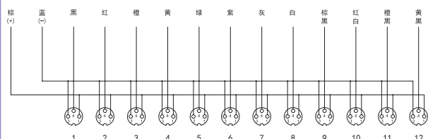
S010-M8-12C S011-M8-12C
