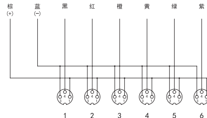
S010-M8-6C S011-M8-6C
