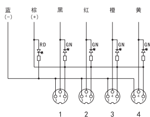
S010-M8-4 S011-M8-4
